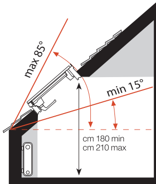
Pendiente mínima y máxima de colocación
