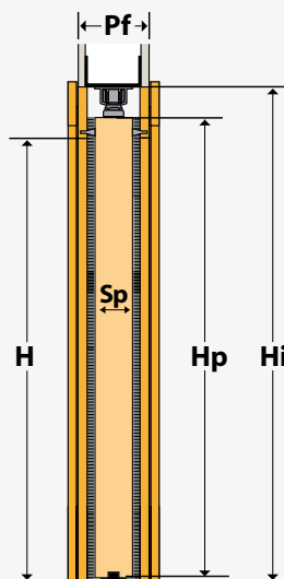
SECCIÓN
