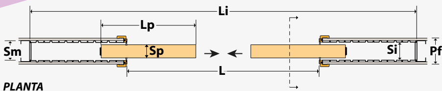
PLANTA
